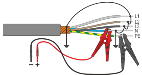
Fig. 3.2. Medición del cable apantallado
